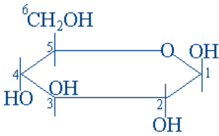
Alfa-D-Glucopiranososa
